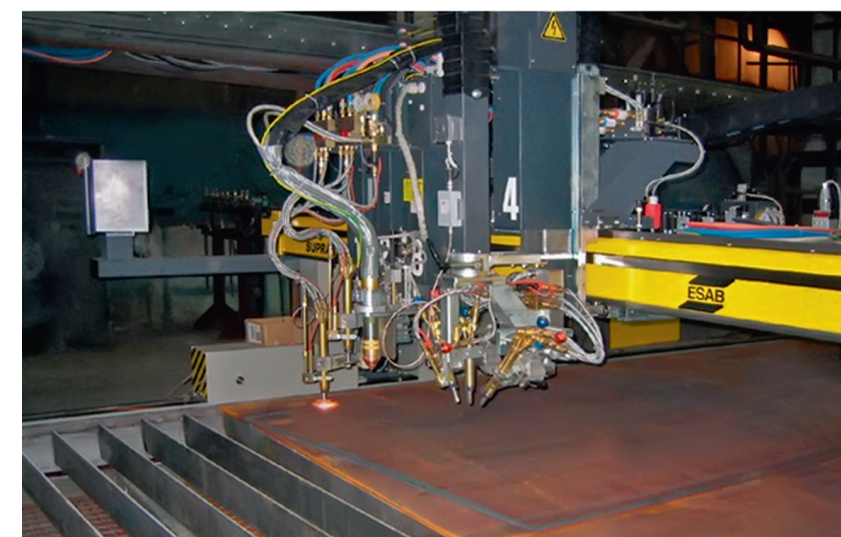
Машина газоплазменной резки.
